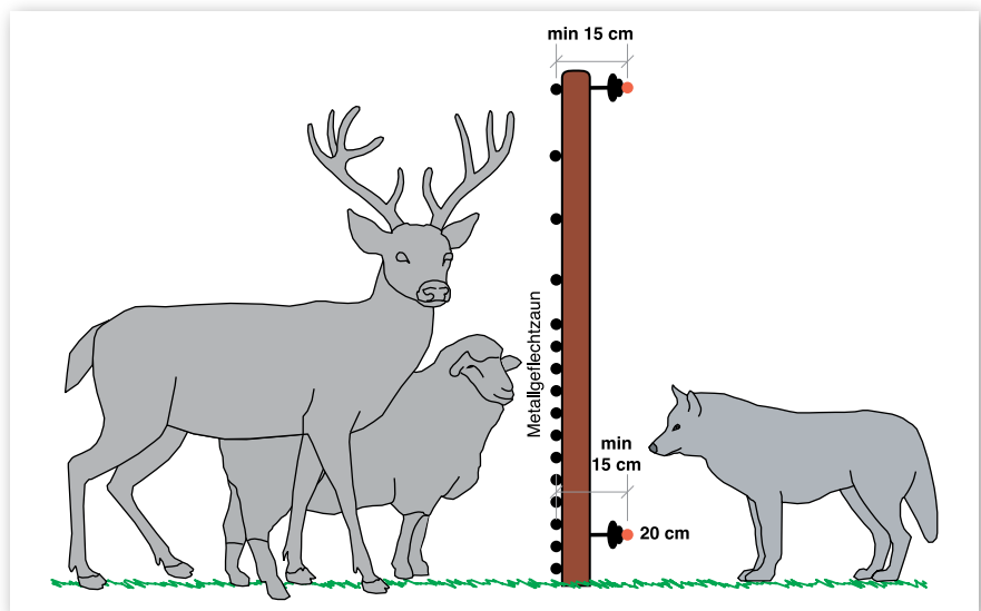
Abbildung 19: Absicherung eines Stabilzäunes mit zwei stromführenden Leitern (© G. Herkert)
