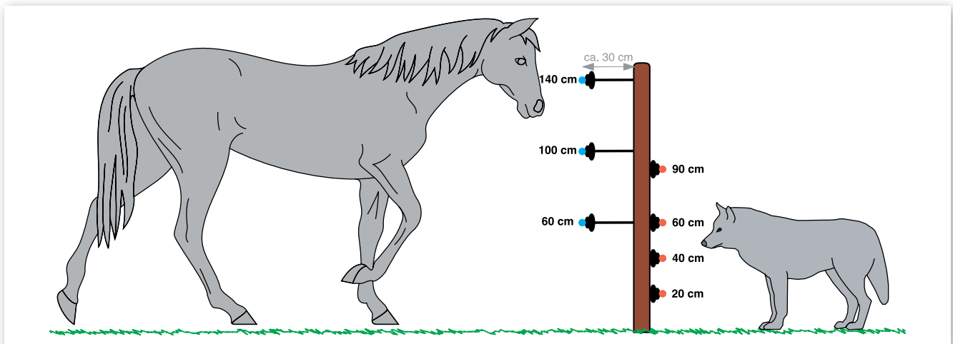
Abbildung 16: Zaunleiter auf Wolfseite am Pfahl (© G. Herkert)
